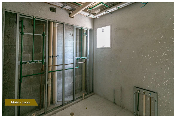
Foto 2 – Tubulações hidráulicas e de gás em unidade.
