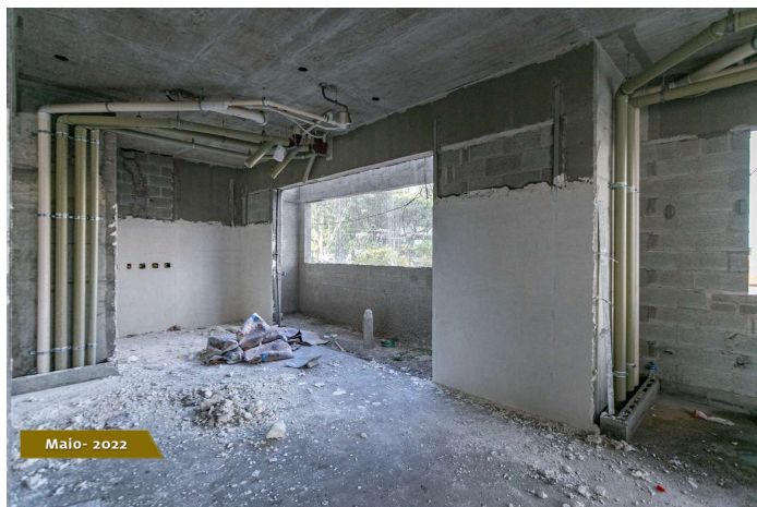
Foto 3 - Tubulações hidráulicas
